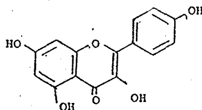
[VI] Kaempferol
