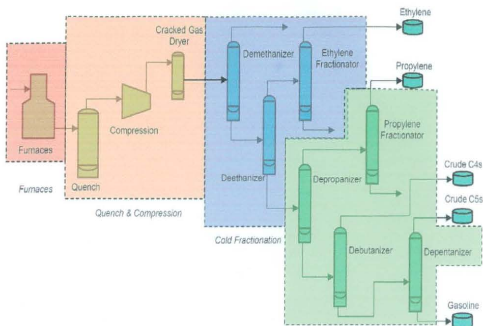
Figura 1 – Fluxograma típico de uma planta de olefinas. (ref. 2)
