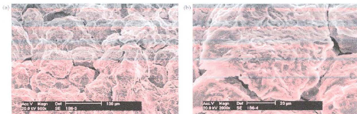
Figura 8 – Superfície de fratura na solda circunferencial, mostrando a natureza intergranular e ramificada das trincas. 1
