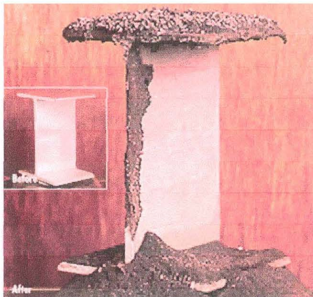
Figura 1 – Efeito corrosivo do mercúrio sobre uma coluna de alumínio.
