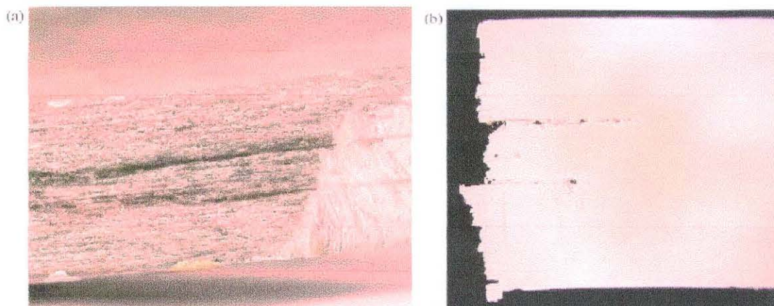
Figura 3 – (a) Fotografia mostrando a superfície da fratura longitudinal e das fraturas de delaminação. (b) secção transversal da fratura após polimento mostrando a natureza e o comprimento da trinca. 1
