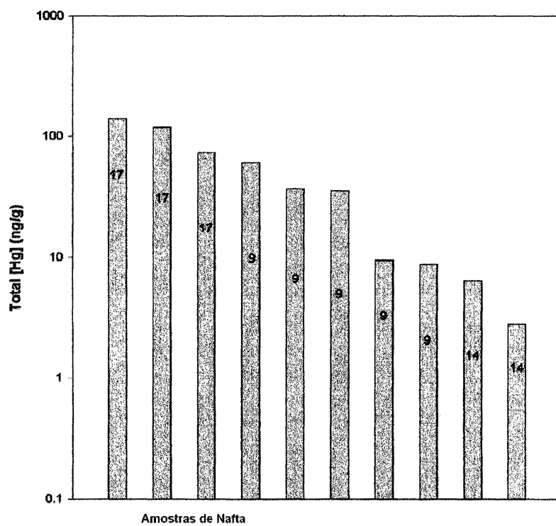
Figura 2. Concentração total de mercúrio em amostras de nafta. (ref. 4)
