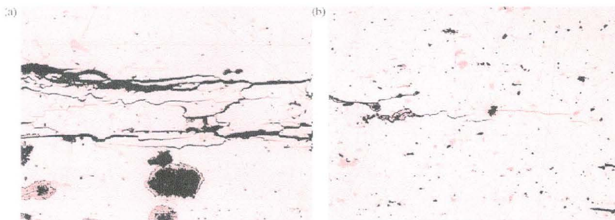
Figura 4 – Secção mostrando as múltiplas trincas próximas da superfície da fratura longitudinal (a) e próximo do fim da fratura por delaminação (b) (aumento de 165 X). 1
