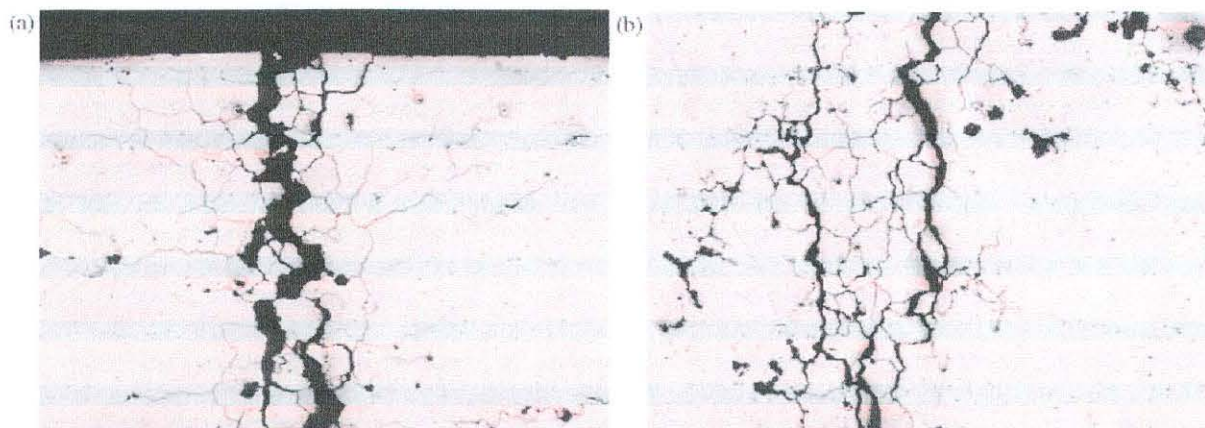
Figura 7 – Trincas na superfície externa da solda circunferencial (a) e no interior dela (b), ilustrando fratura intergranular ramificada (aumento de 141X). 1
