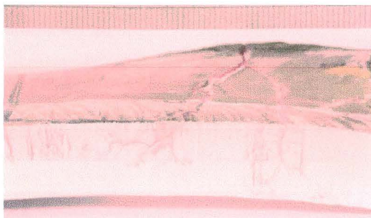
Figura 6 – Vista macroscópica de uma secção da solda cicunferencial, mostrando fratura intergranular pronunciada e ramificada. 1
