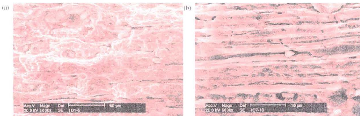
Figura 9 – (a) Superfície de fratura longitudinal no topo de margem elevada e (b) ilustrando fratura lamelar. 1
