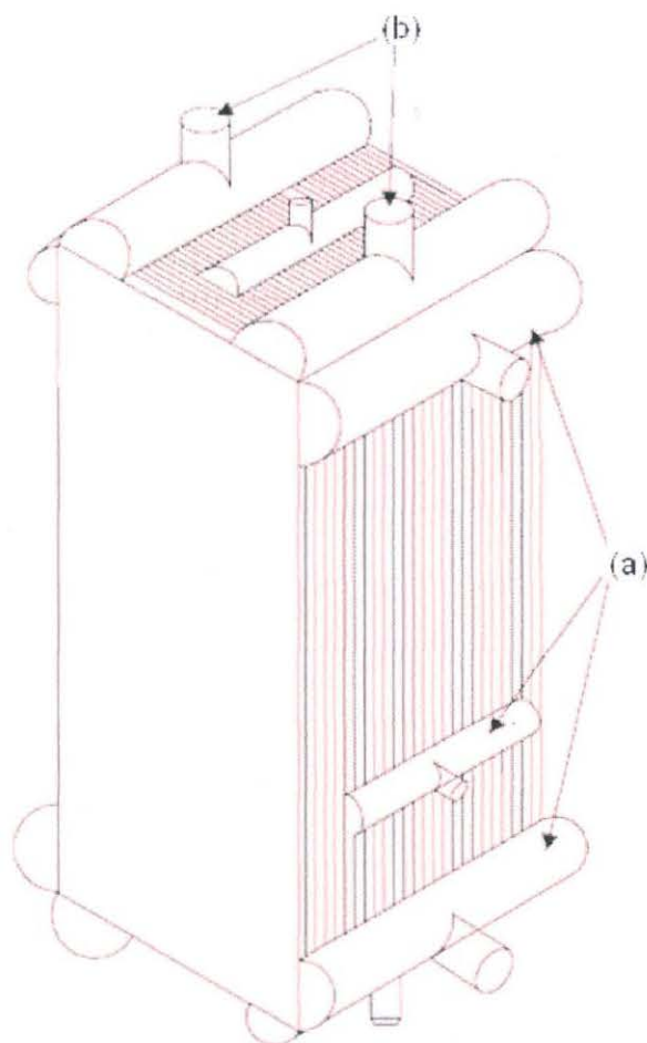
Figura 2 – Vista esquemática de um trocador de calor criogênico mostrando distribuidores (a) e bocais (b). 1
